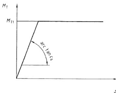
Figure C.1 — Relation M_B - \varphi pour la classe B de raccords orthogonaux
