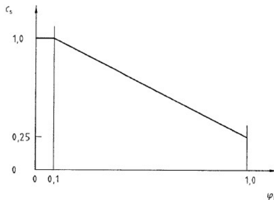
Figure 6 — Coefficient d'emplacement c_{s,i} pour les échafaudages de service montés devant une façade et pour des charges dues à l'action du vent perpendiculaires à la façade
